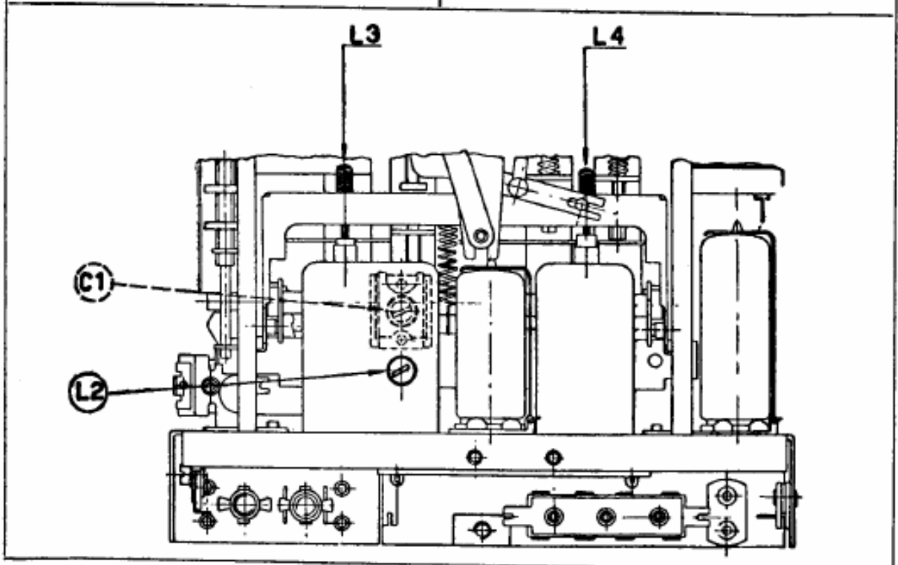
AUTOVOX - Mod. RA 49 prima e seconda serie. Operazioni di allineamento. A 1600 kc regolare C8 (pos. 1,5); a 520 kc regolare L5 (pos. 0,52) poi C2; a 1000 kc regolare prima L4 poi L3 (pos. 1). Ripetere l'allineamento. A 6,1 Mc regolare prima L6 poi L2 (pos. 6,1, a sinistra in alto).
